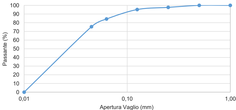
Curva granulometrica MICRO-POZZ PFA Cat. C-N
